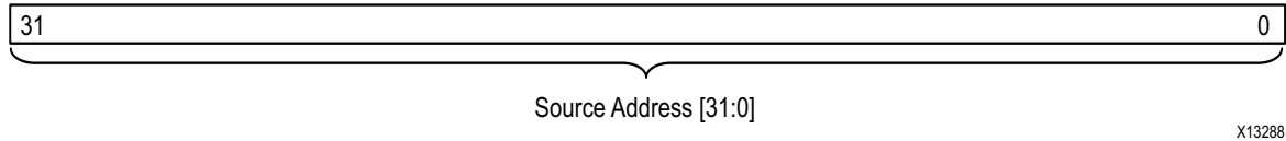
Figure 2-8: SA Register
