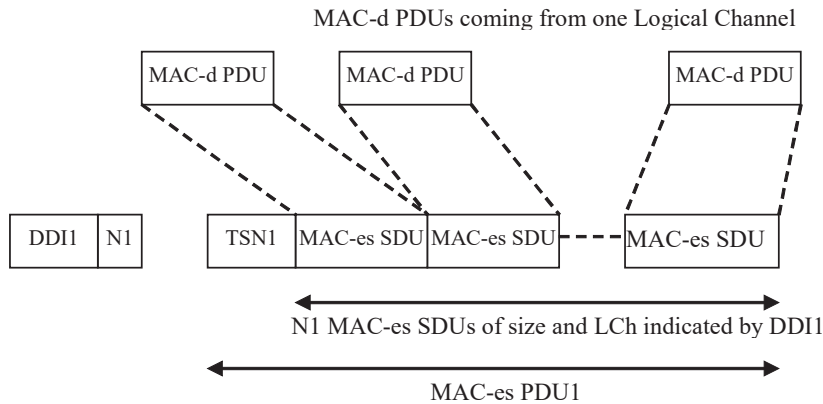
Figure 9.1.5.1 MAC-es PDU
