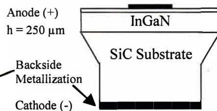
Die Cross Section
