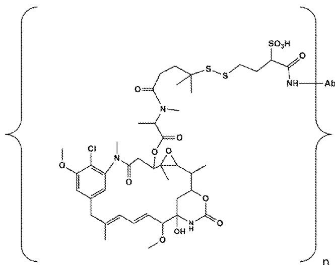
Ab-sulfo-SPDB-DM4
