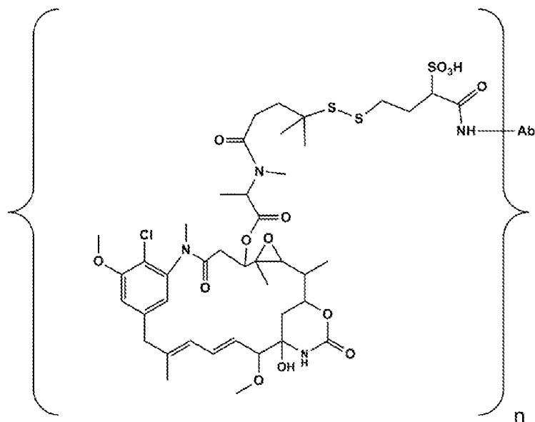
Ab-sulfo-SPDB-DM4
