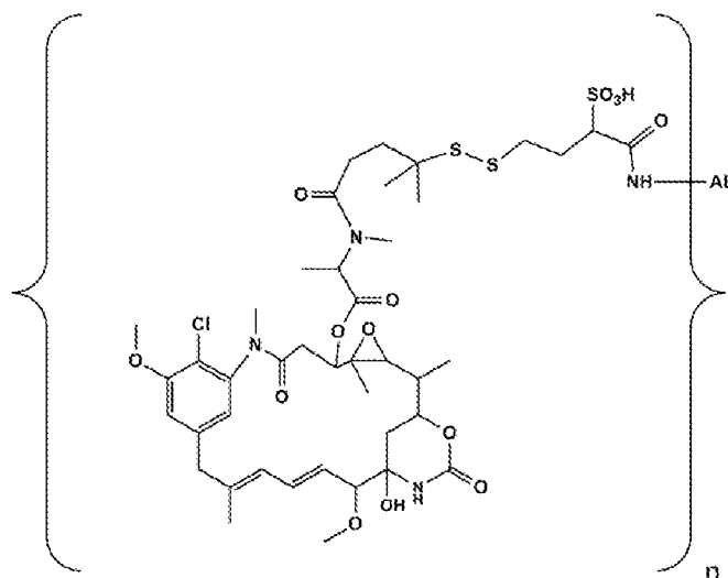
Ab-sulfo-SPDB-DM4
