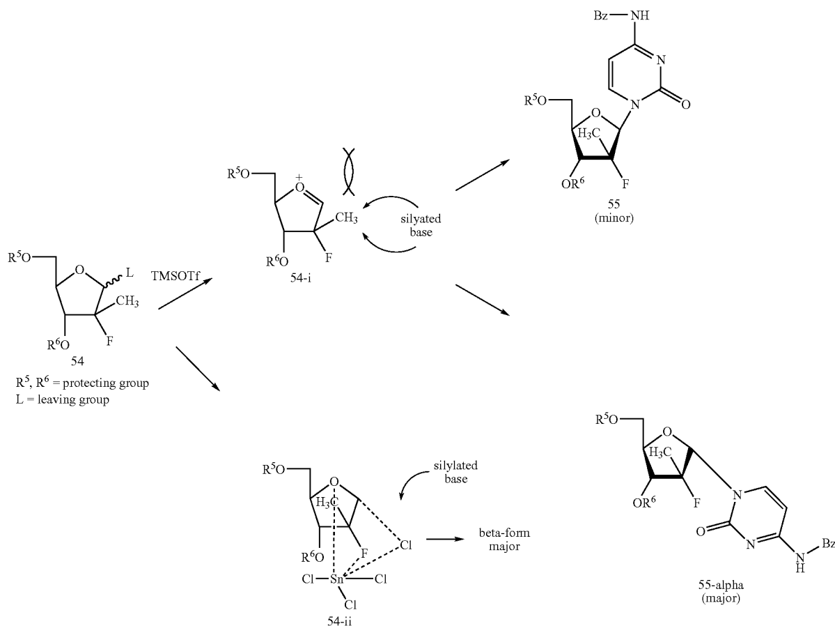
Scheme 10a
