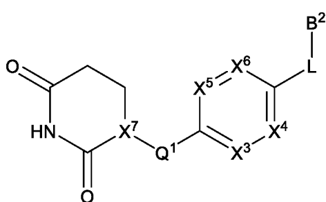
(V); or
