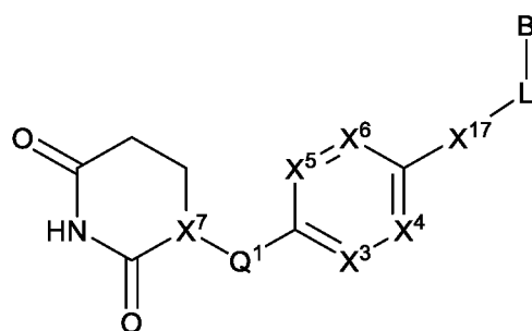
(V); or
