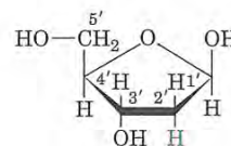
Deoxyribose
