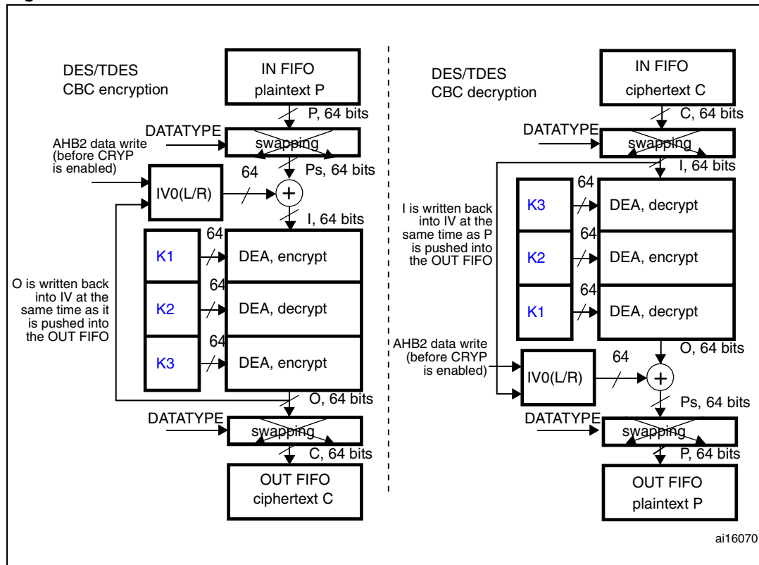
Figure 198. DES/TDES-CBC mode
