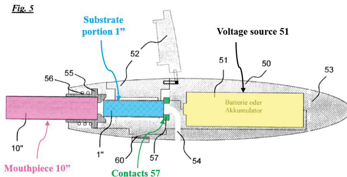
EX1006, FIG. 5.
