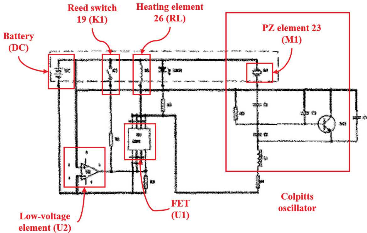
EX1029, FIG. 12.
