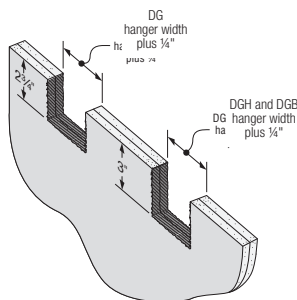
Drywall Notches
