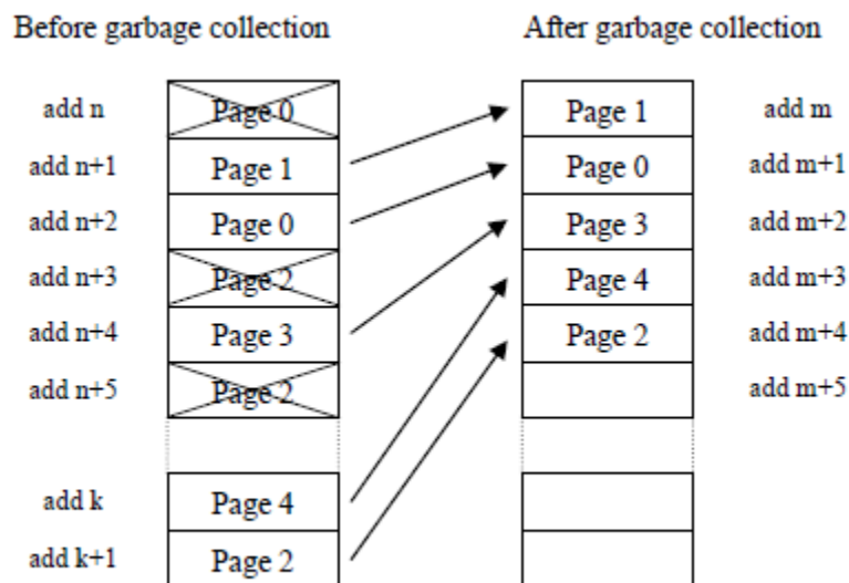
Fig. 17.7. Garbage collection
