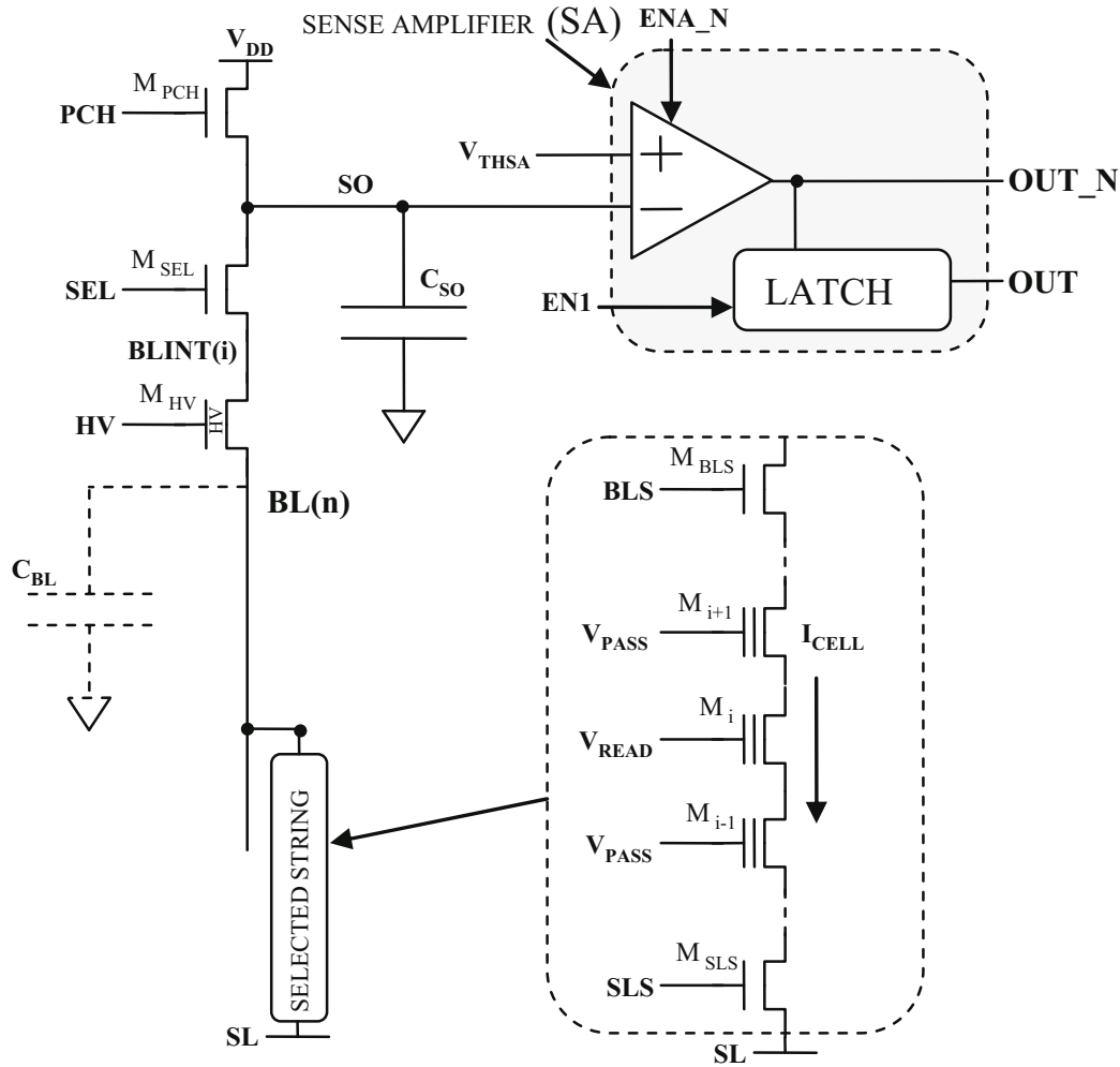
Fig. 6.26 ABL sense amplifier
