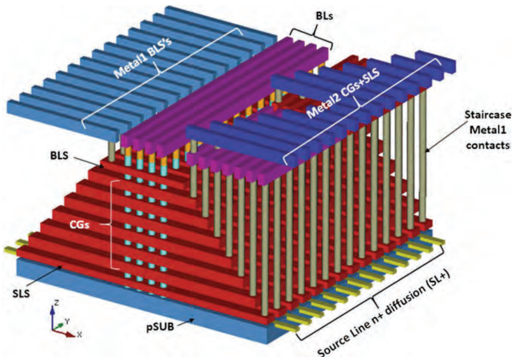
Fig. 5.12 TCAT NAND Flash array
