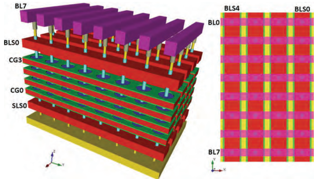
Fig. 5.19 C-FG NAND Flash array
