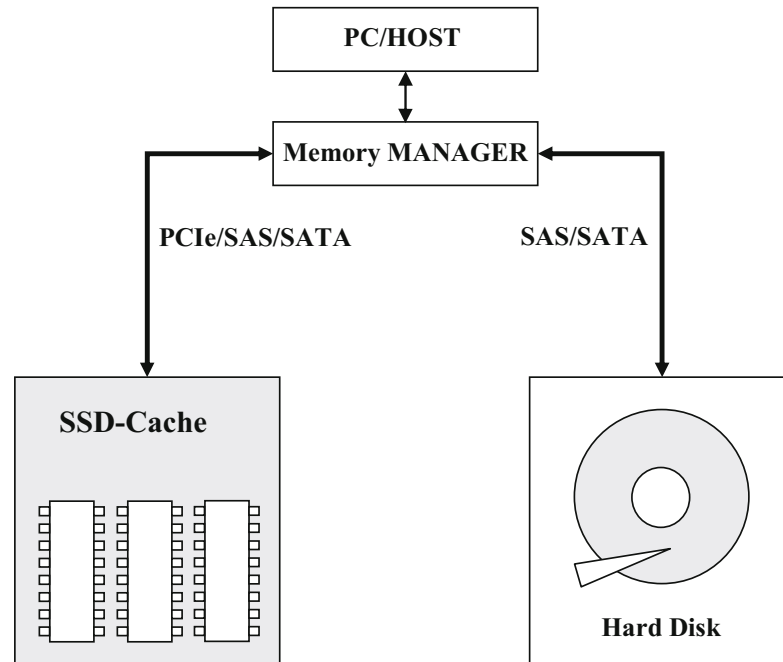
Fig. 3.7 SSD-Cache
