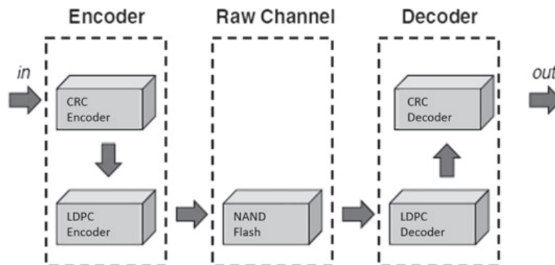
Fig. 11.30 Concatenation LDPC + CRC
