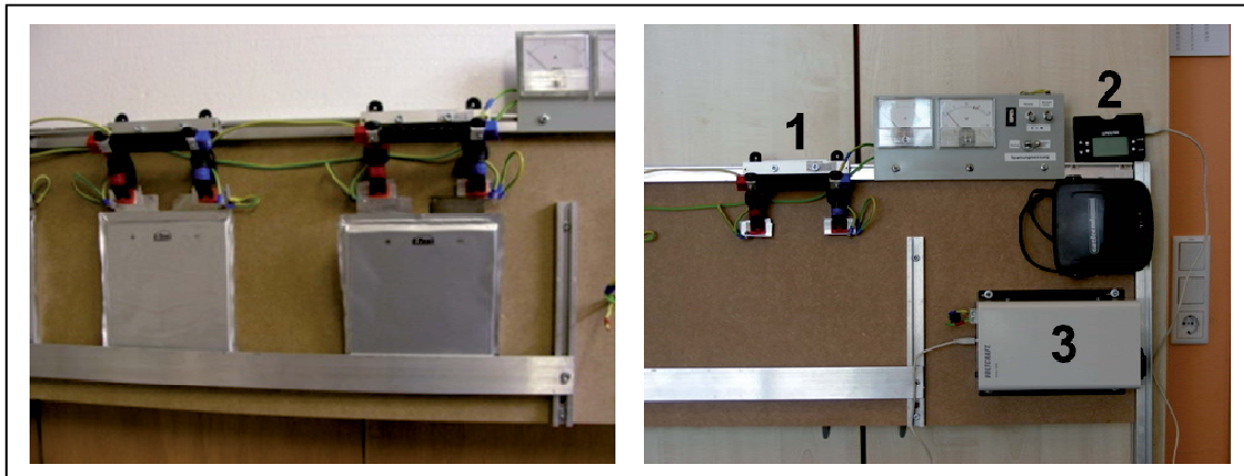
Abbildung A-24: Aktuelle Zellentladung und Greiferlösung
