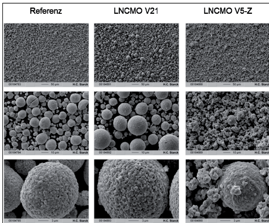
Abbildung C-3: REM-Aufnahmen des Referenzmaterials und der LNCAO-Materialien aus recycelten Lösungen bei 200-, 1.000- und 5.000-facher Vergrößerung
