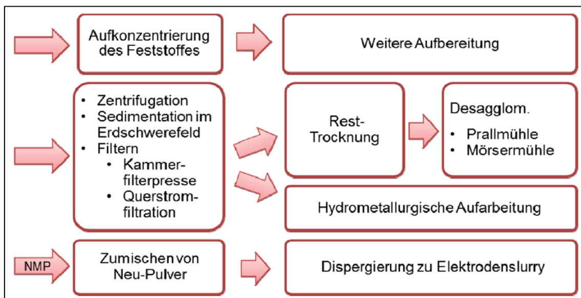
Abbildung B-29: Aufkonzentrierung und weitere Aufarbeitung nach der nasschemischen Separation
