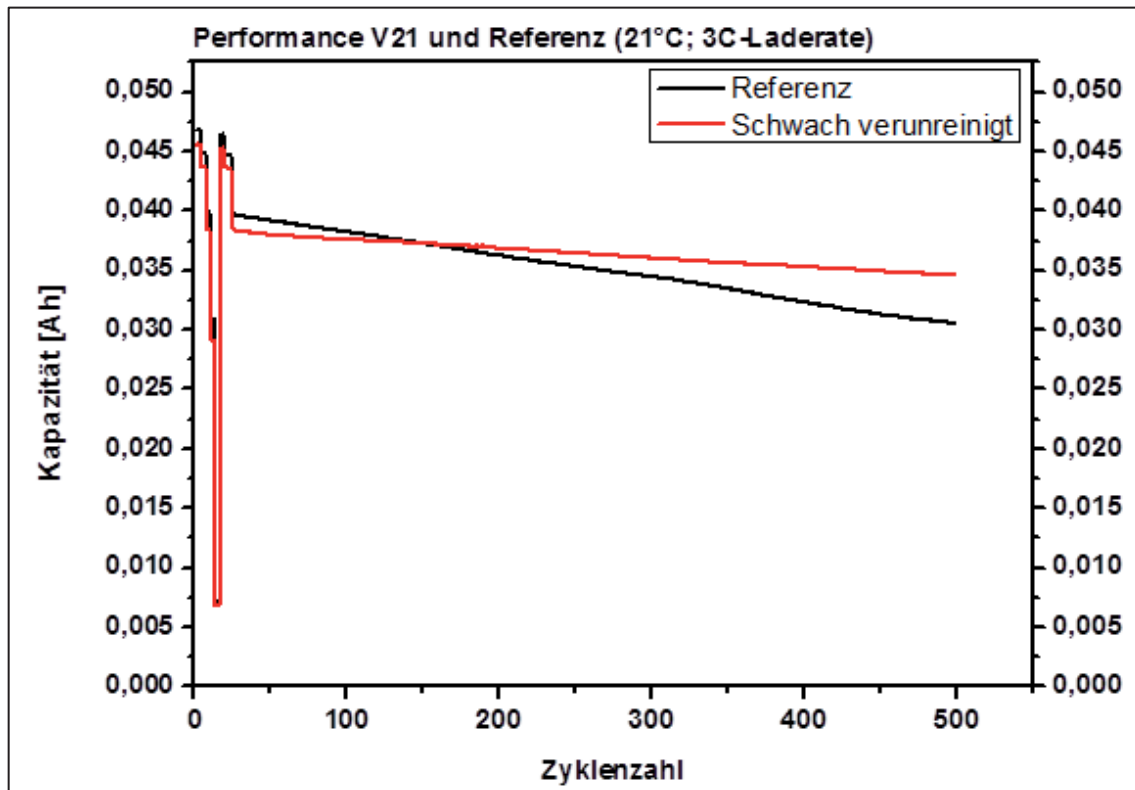
Abbildung C-14: Performance V21 und Referenz
