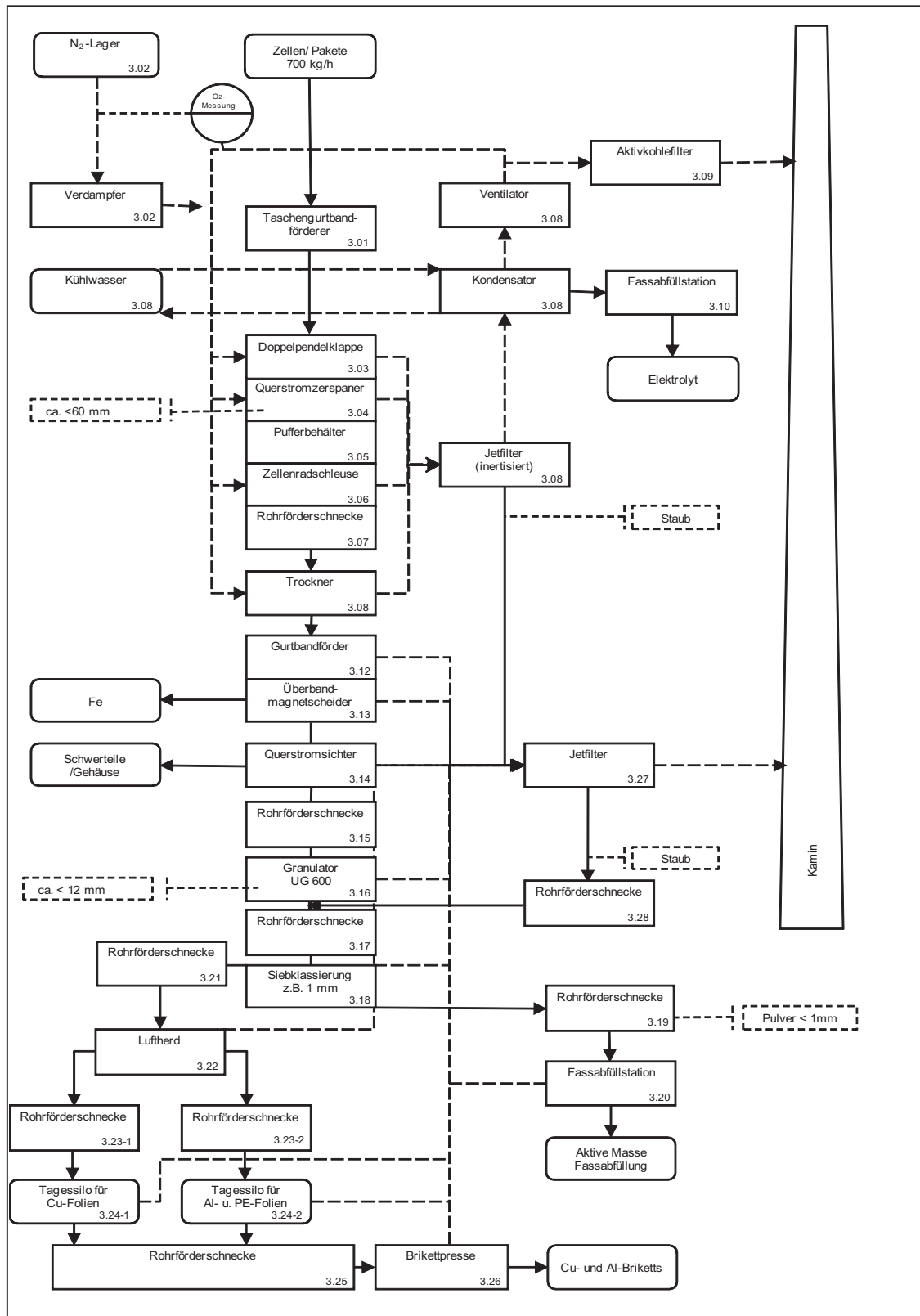
Abbildung G-1: Verfahrensfließbild mechanische Aufbereitung
