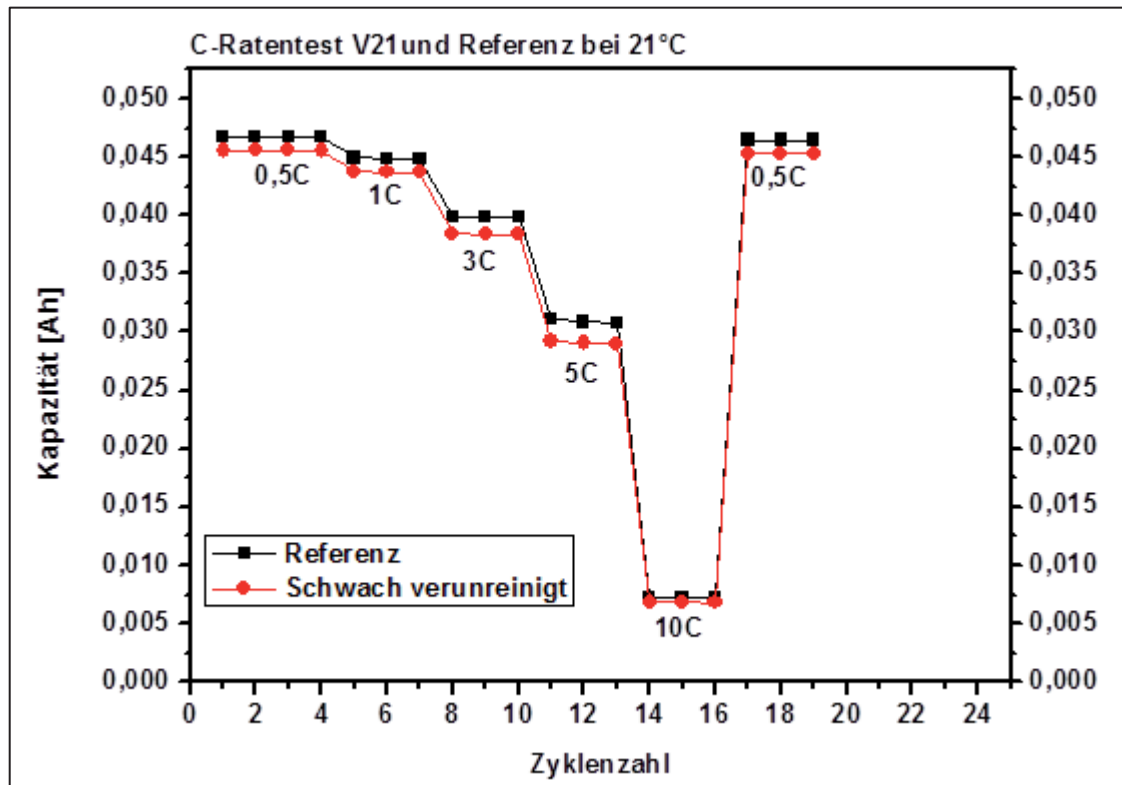
Abbildung C-13: C-Ratentest V21 und Referenz
