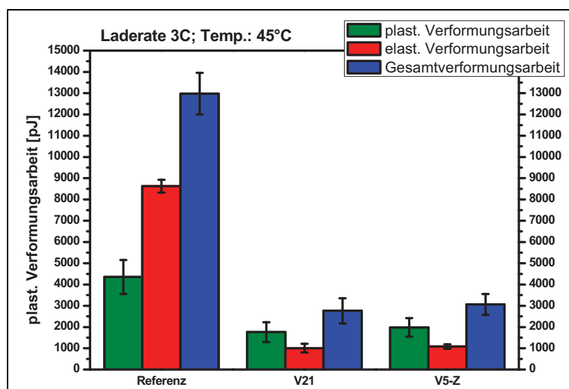
Abbildung D-23: Nanoindentation von Recyclingmaterial. Laderate 3C, Temperatur 45°C
