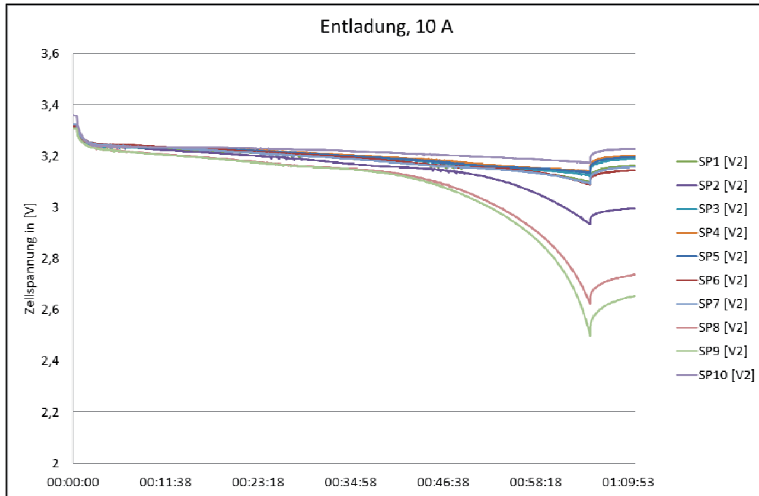
Abbildung D-5: Entladung der zu charakterisierenden Standardzellen
