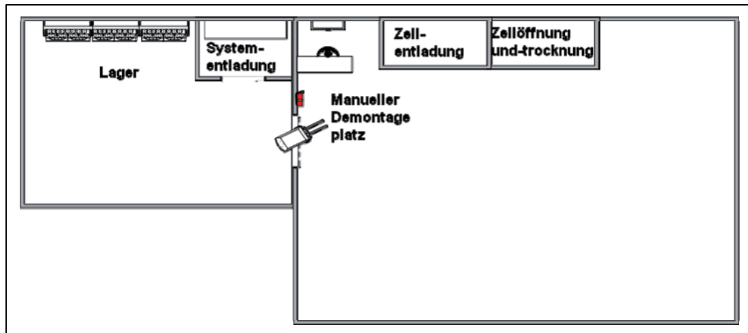
Abbildung B-11: Layout eines Demontagesystems für Szenario „2015 realistisch“
