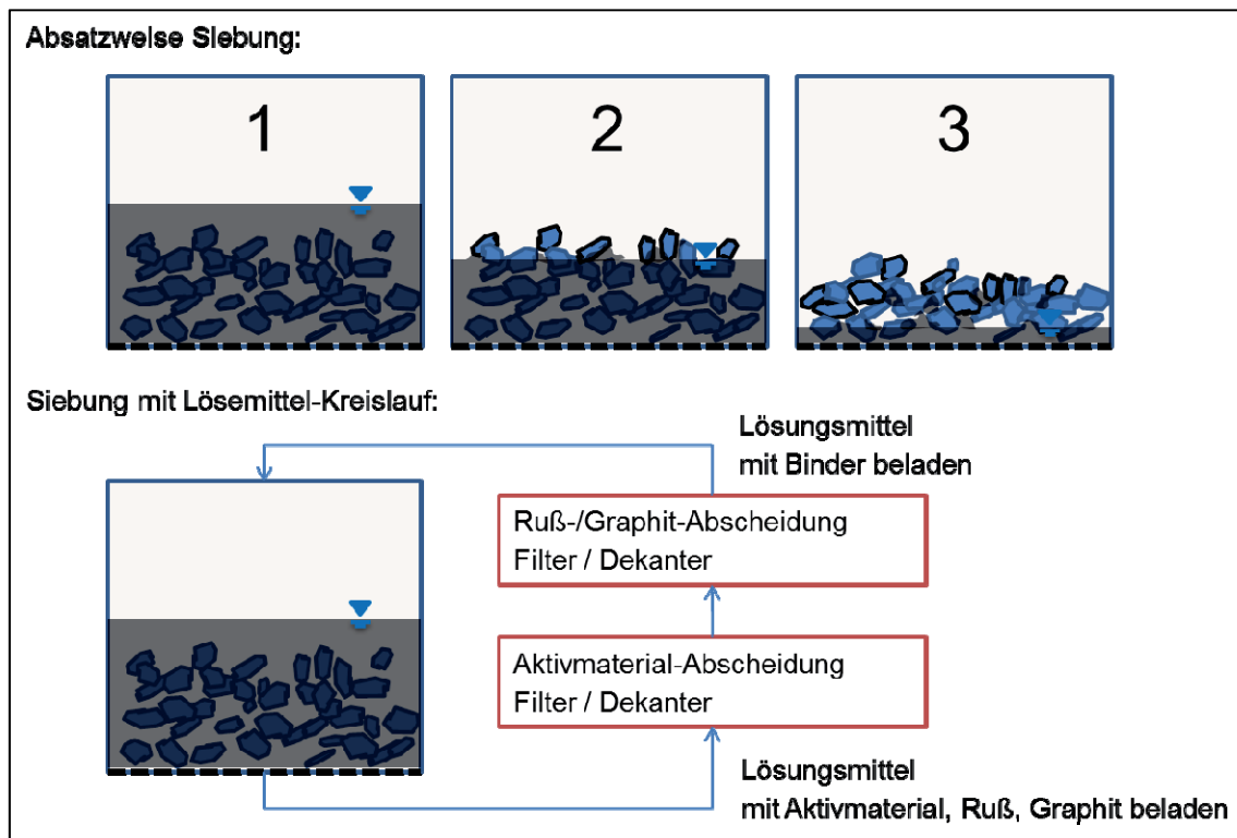
Abbildung B-26: Wirkmechanismus Batch-Filtration (oben), Fahrweise mit Lösungsmittel-Kreislauf (unten)
