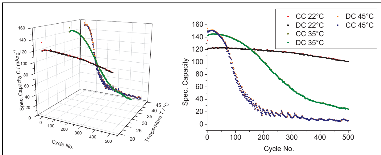
Abbildung D-3: Temperaturmatrix 1CCC mit LiBF4 in EC/DMC
