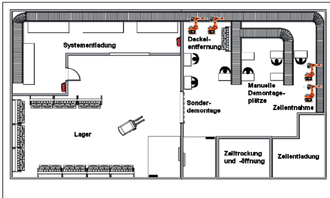
Abbildung B-12: Layout eines Demontagesystems für Szenario „2030 realistisch“
