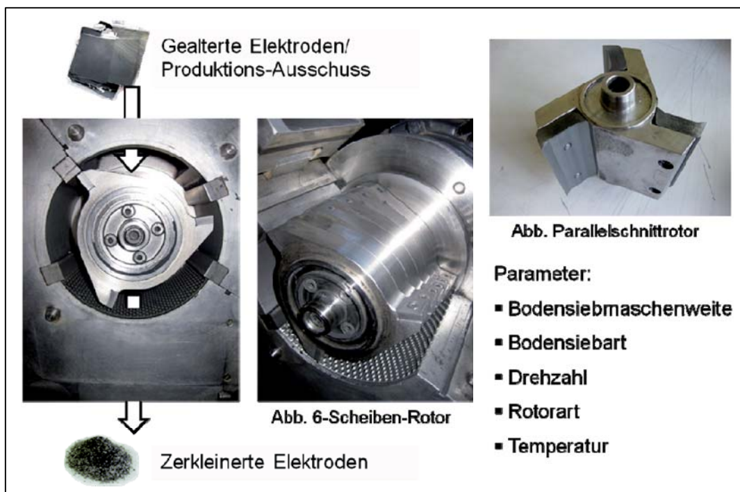
Abbildung B-22: Mechanische Separation in der Schneidmühle
