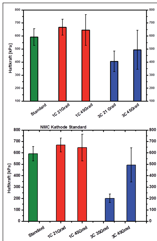
Abbildung D-13: Haftkraftmessung an zyklisierten Zellen (Standard)
