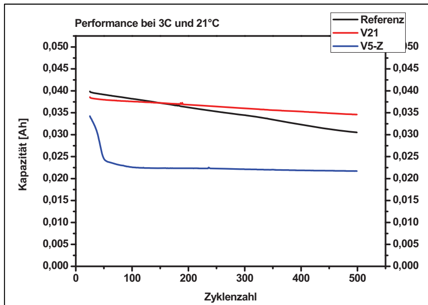
Abbildung D-18: Performance NMC bei 21°C und 3C
