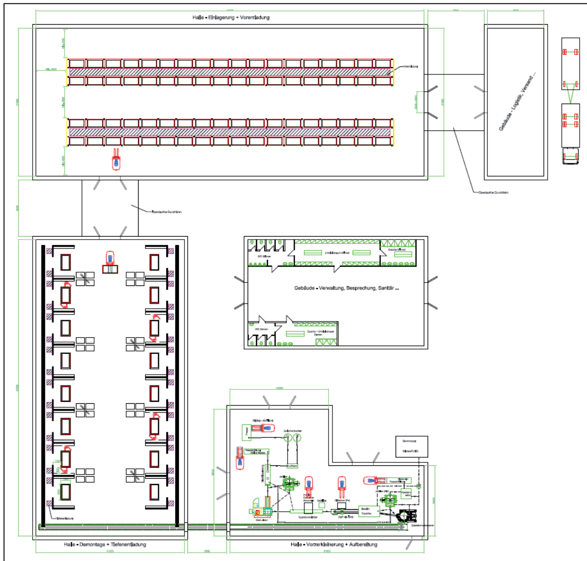
Abbildung G-2: Layout der Aufbereitungsanlage für Lithium-Ionen-Batterien
