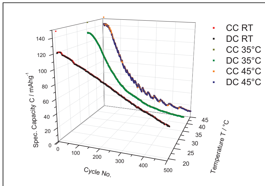
Abbildung D-4: Temperaturmatrix 3CCC mit LiBF4 EC/DMC
