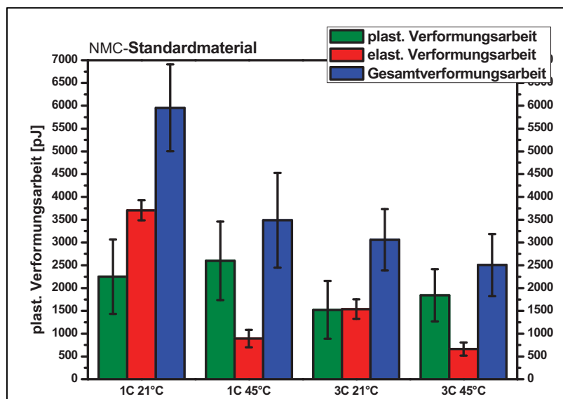
Abbildung D-14: Nanoindentationsmessungen an NMC-Standardmaterial
