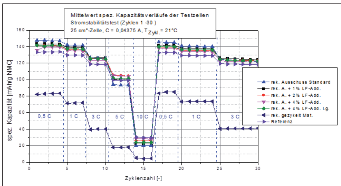
Abbildung C-9: Strombelastbarkeitstest rekonditionierter Materialien
