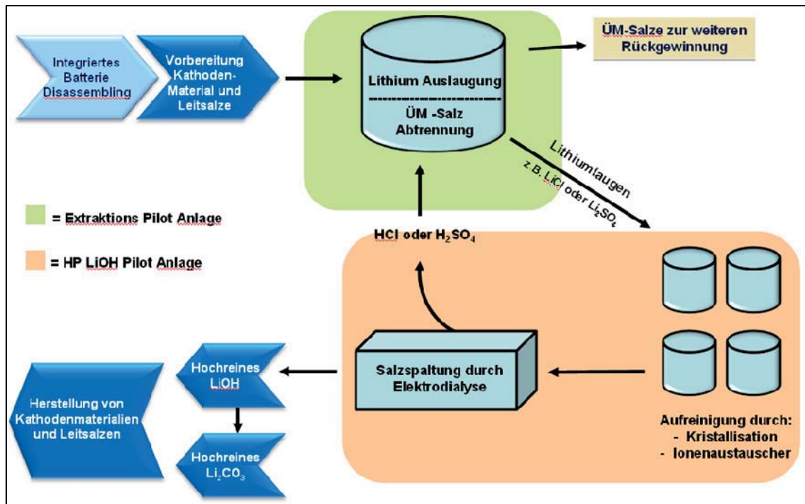
Abbildung B-30: Projektschema Hydrometallurgisches Batteriematerialrecycling
