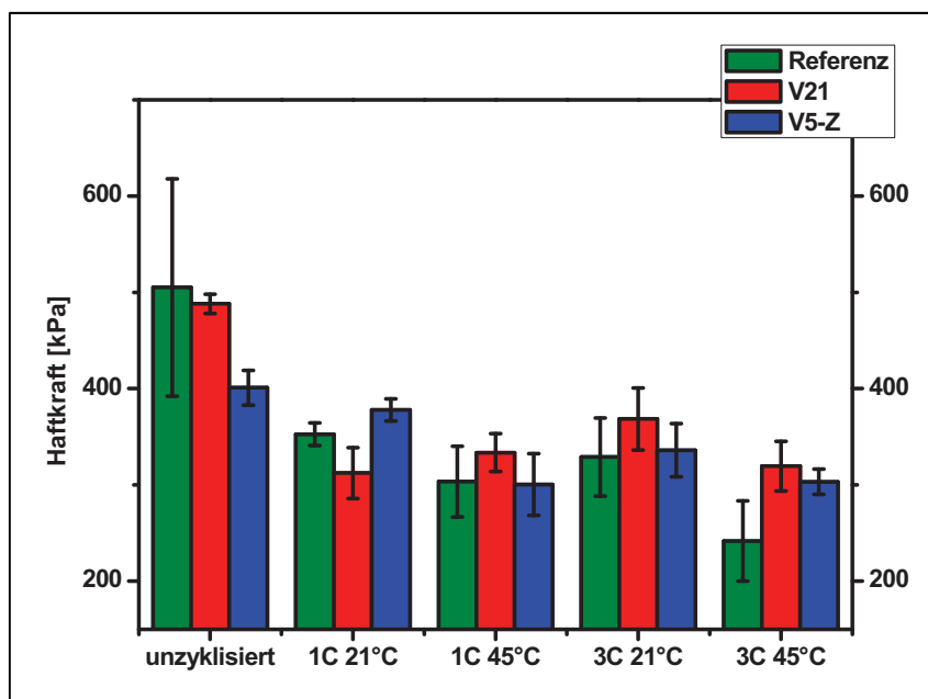
Abbildung D-20: Haftkraftuntersuchung von NMC-Material bei unterschiedlichen Laderaten und Temperaturen
