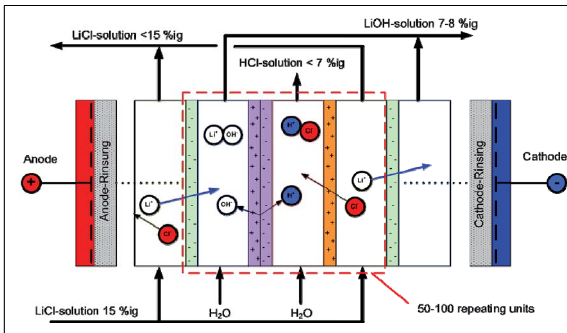
Abbildung B-34: Funktionsweise einer Elektrodialyse mit bipolarer Membran
