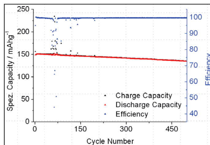
Abbildung D-1: Zyklisierungskurve von LiFePO 4 bei 40°C
