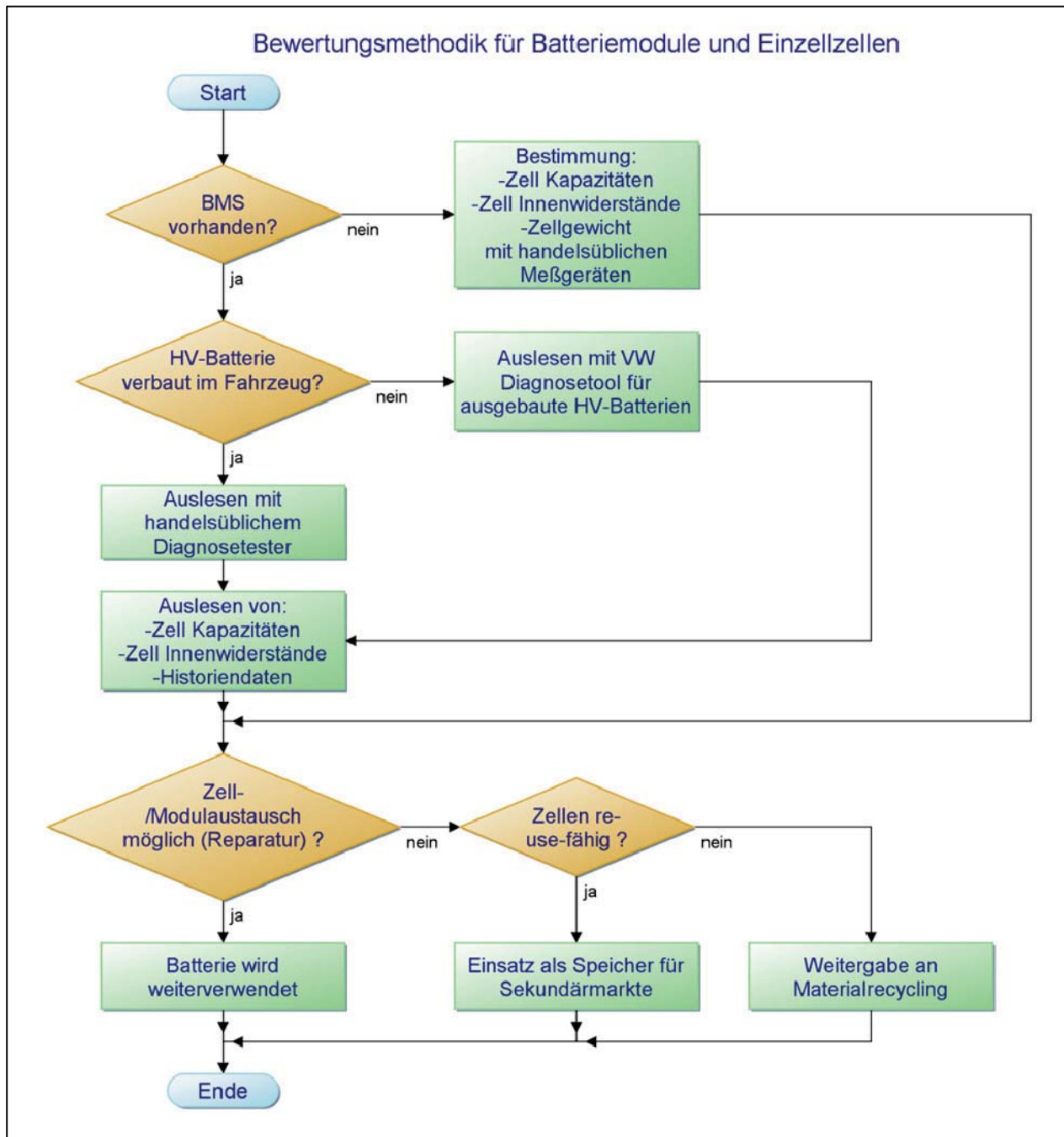
Abbildung A-22: Prüfschema technische Zustände Module und Zellen
