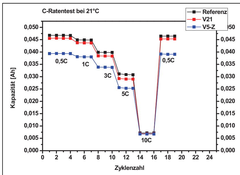
Abbildung D-16: C-Ratentest NMC bei 21°C
