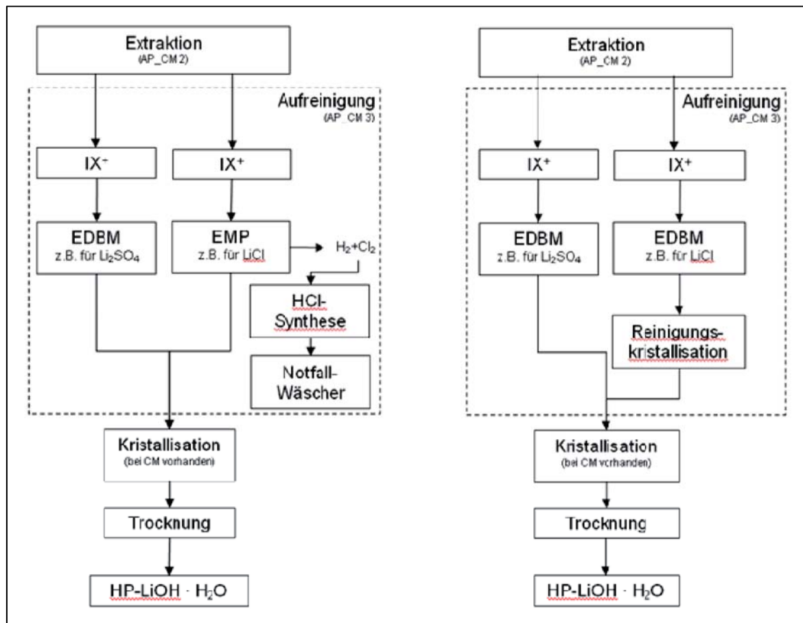
Abbildung B-35: Ursprüngliches und verbessertes Verfahrenskonzept
