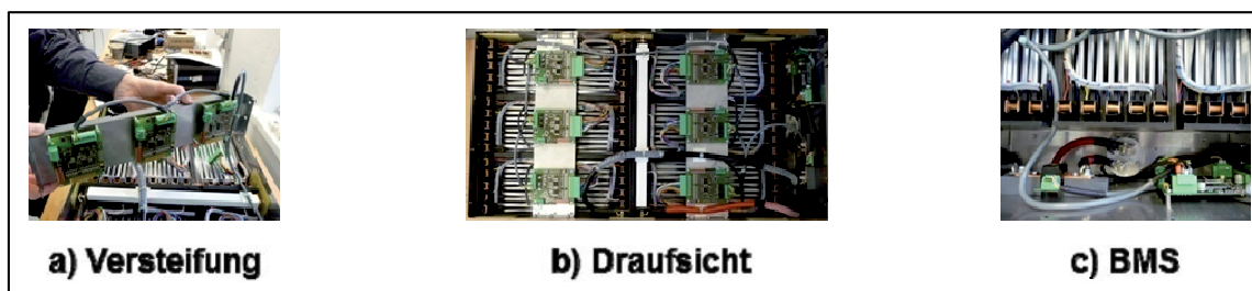
Abbildung B-1: Eindrücke der Testdemontage des Batteriesystems A
