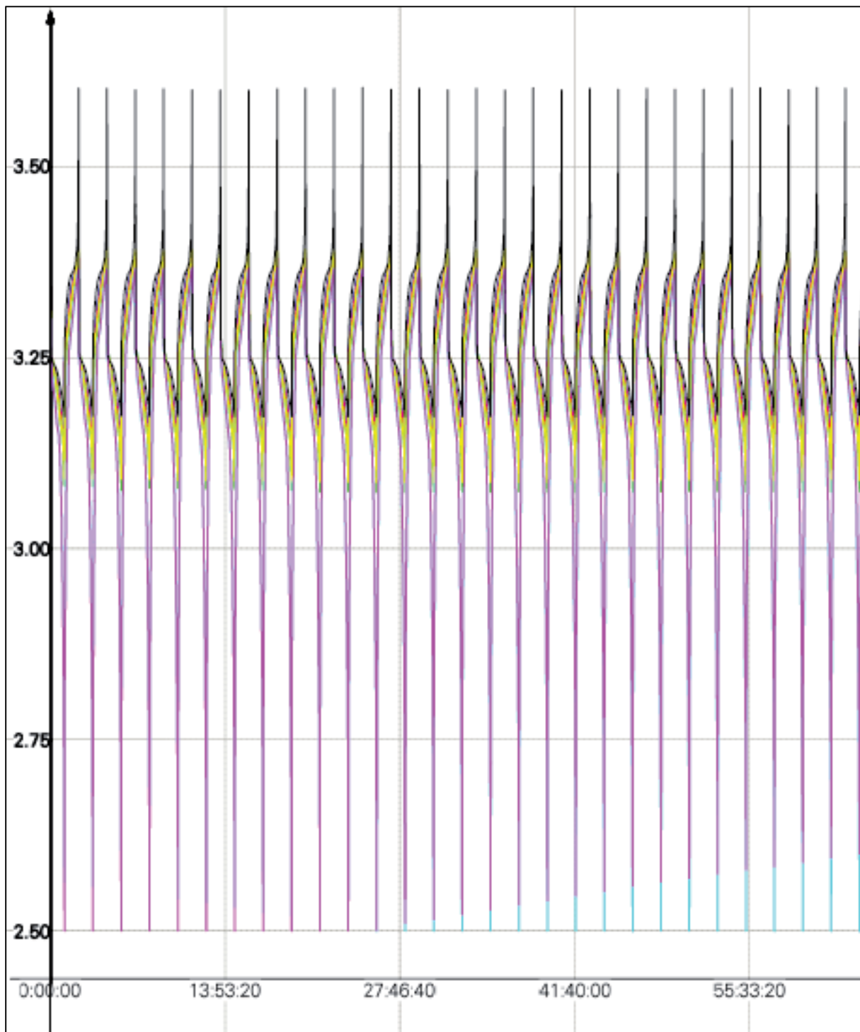
Abbildung D-9: Zellspannungsverlauf während der Zyklisierung
