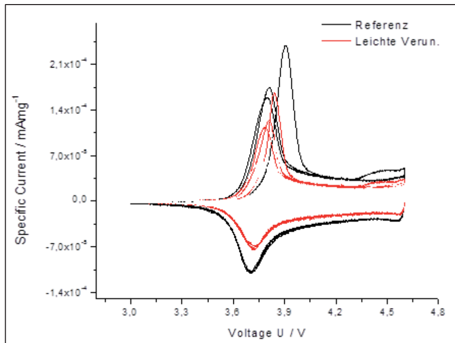
Abbildung C-12: CV Test
