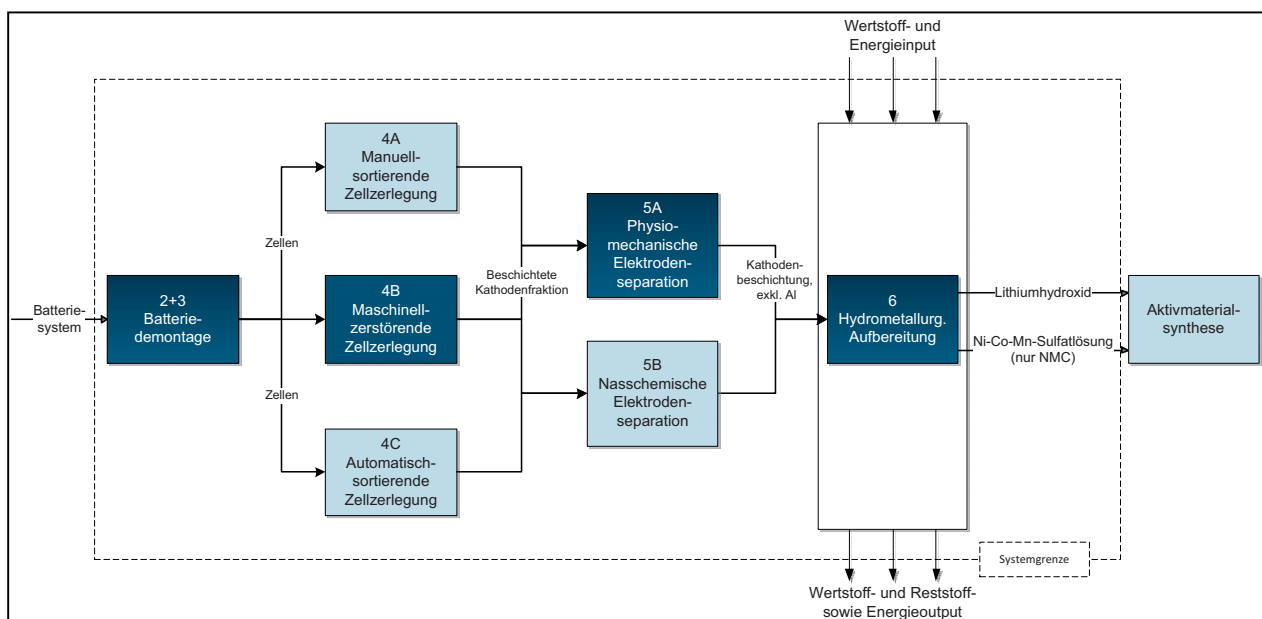
Abbildung E-2: LithoRec-Prozesskette mit alternativen Prozesspfaden
