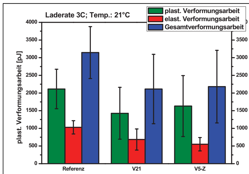
Abbildung D-22: Nanoindentation von Recyclingmaterial. Laderate 3C, Temperatur 21°C
