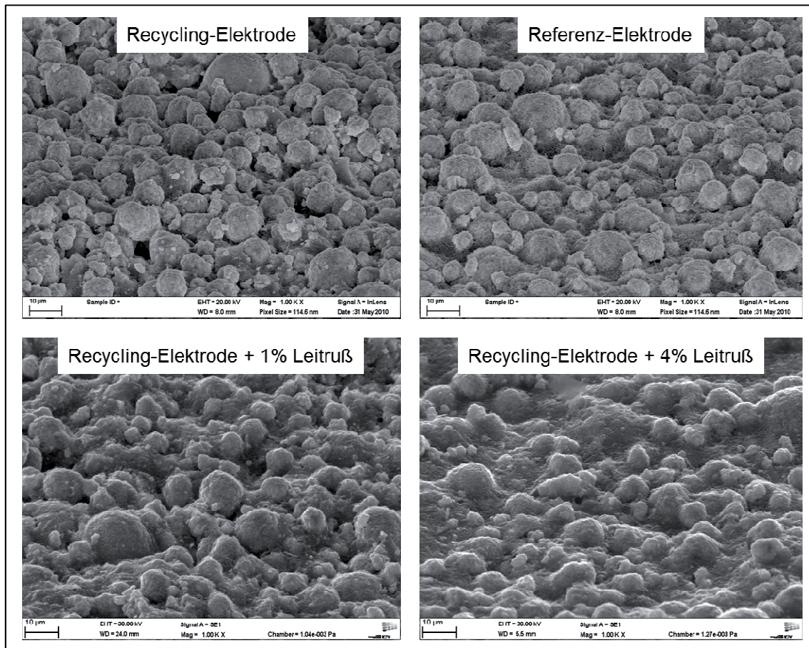
Abbildung C-10: Sekundärelektronenmikroskopische Aufnahmen der Oberfläche von rekonditionierten Elektroden, Winkel 60°(Quelle: IPC-WWU und iPAT-TUBS)
