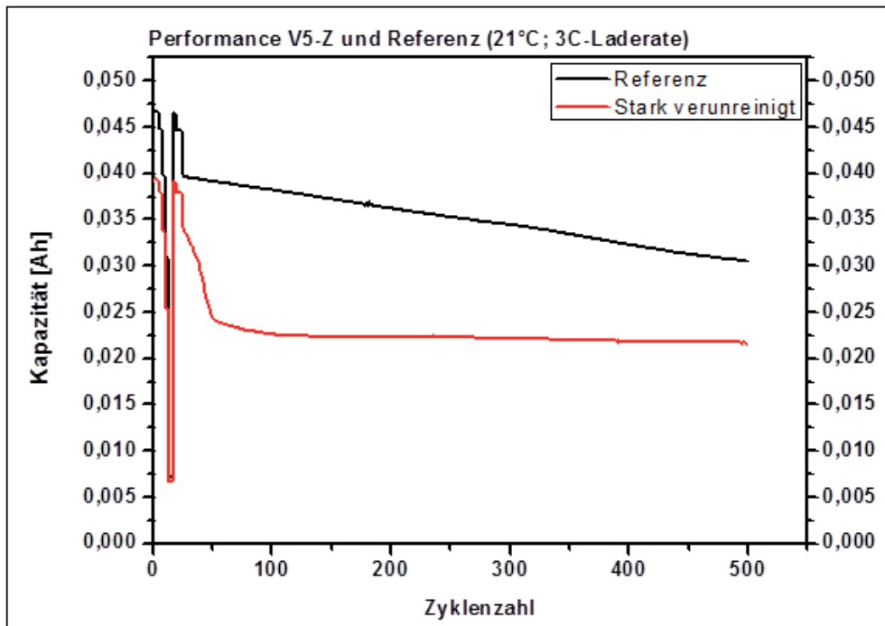
Abbildung C-20: Performance V5-Z und Referenz
