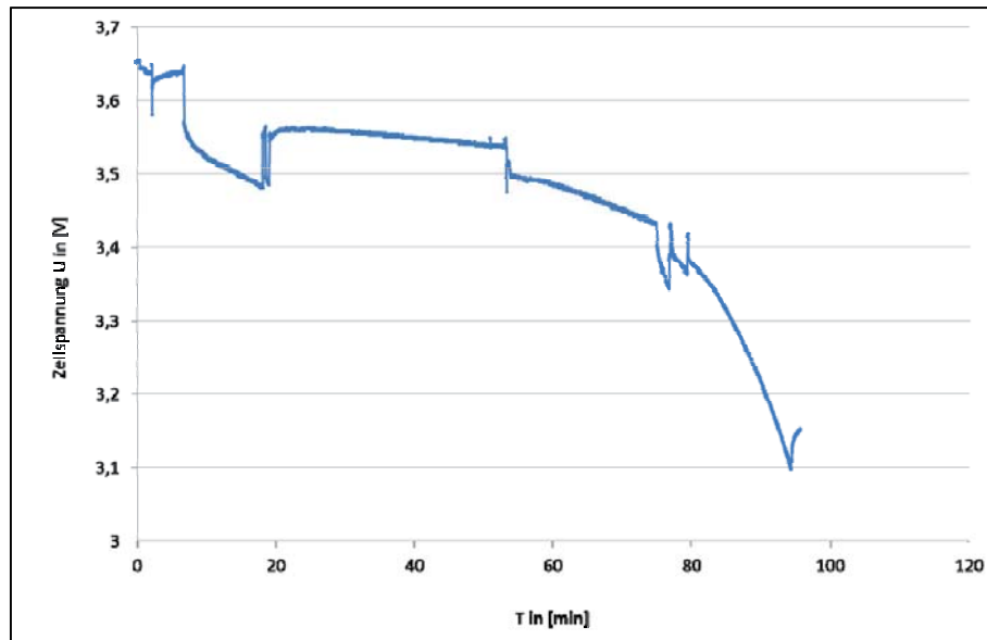
Abbildung A-26: Zellspannungsverlauf während der Entladung
