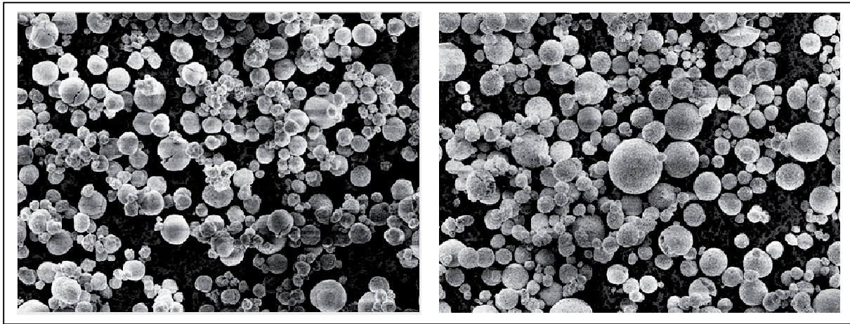
Abbildung C-11: Referenz (links) und leichte Verunreinigung (rechts)
