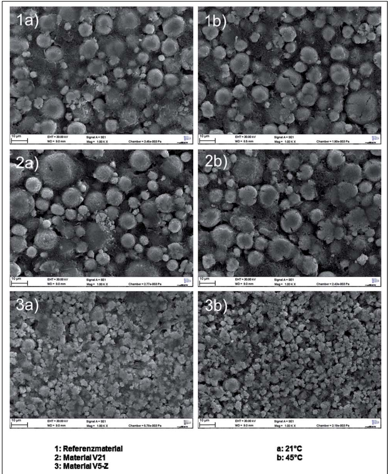
Abbildung D-21: SEM-Aufnahmen von NMC Recyclingmaterial bei 1C-Laderate
