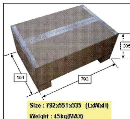
Abbildung A-11: Einwegkartonverpackung Sanyo Batteriesystem für Audi Q5
