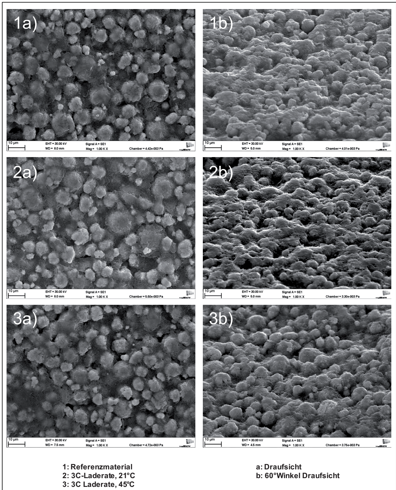
Abbildung D-15: SEM-Aufnahmen von NMC Standardmaterial
