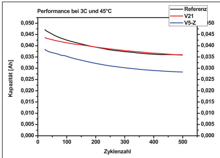
Abbildung D-19: Performancetest NMC bei 45°C und 3C
