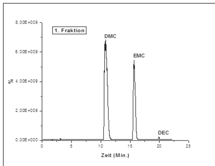
Abbildung B-19: Untersuchung der 1. Fraktion des Destillationsprozesses mittels GC-MS (IPC-WWU)
