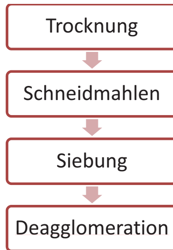
Abbildung B-21: Prozessfließbild der Trockenen Separation
