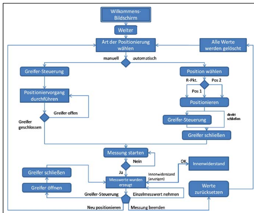
Abbildung B-15: Bedienkonzept des Greifersystems
