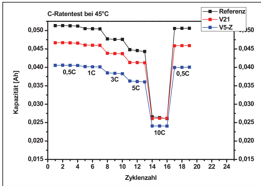
Abbildung D-17: C-Ratentest NMC bei 45°C
