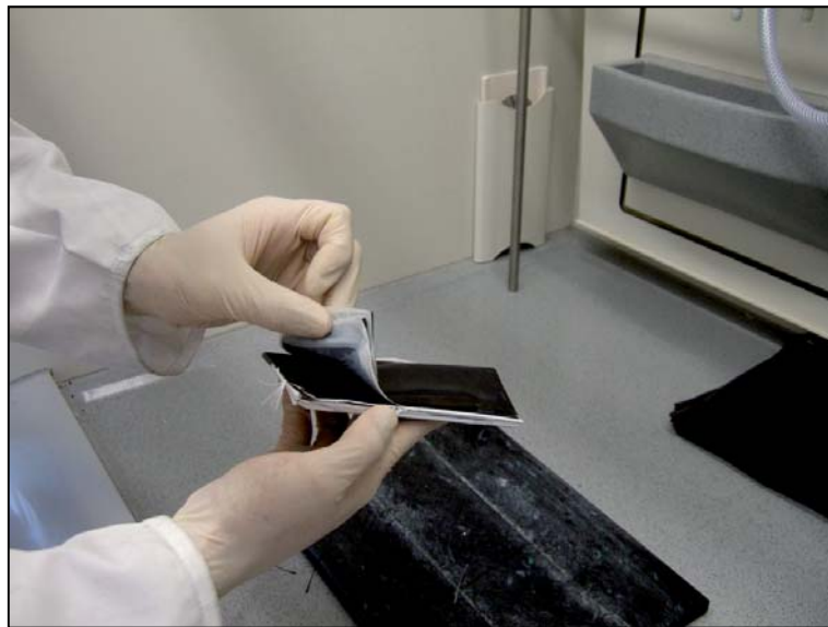
Abbildung B-18: Elektroden-Stack (IPC-WWU)
