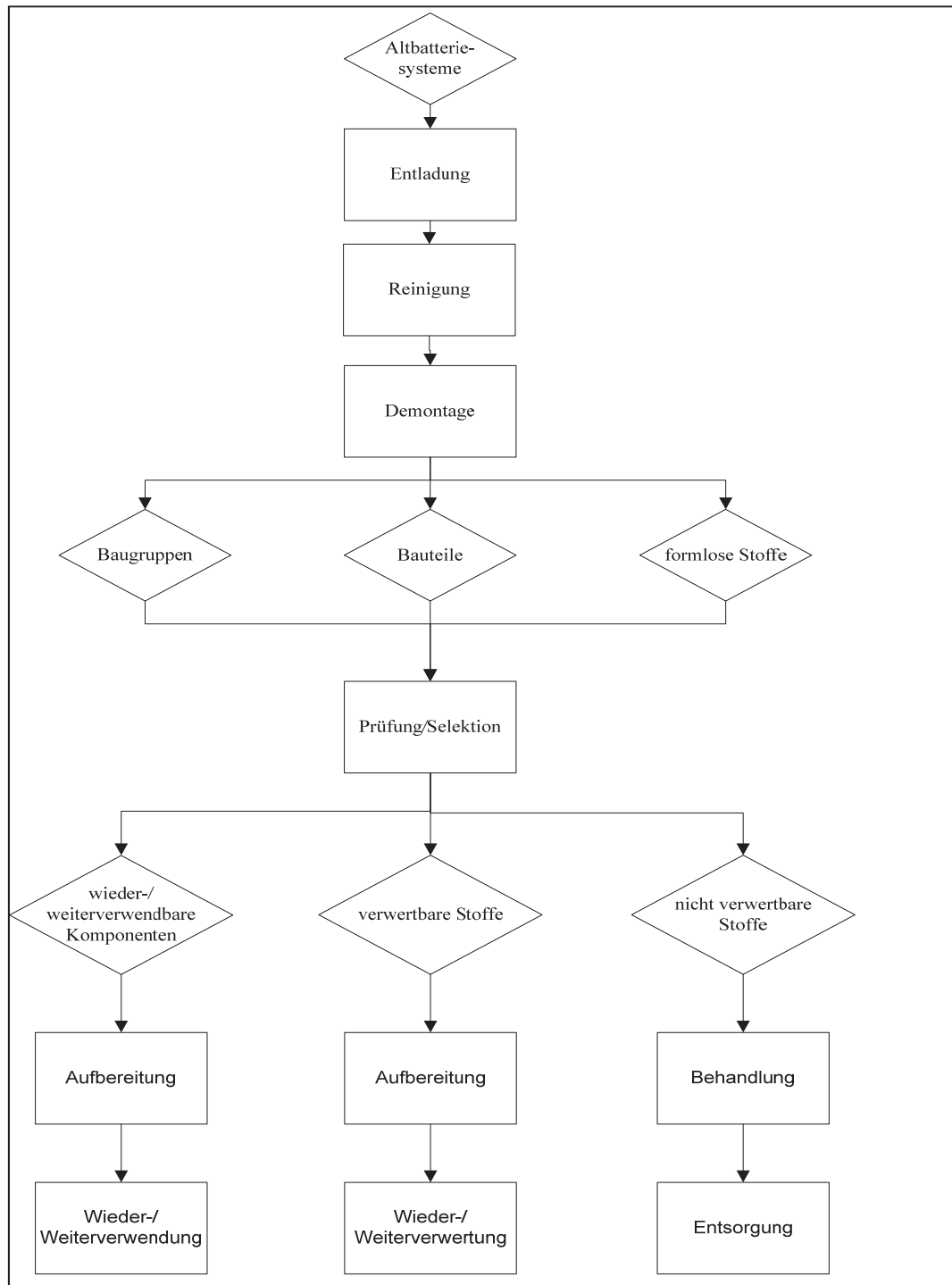
Abbildung B-10: Schema der allgemeinen Demontage von Batteriesystemen 14
