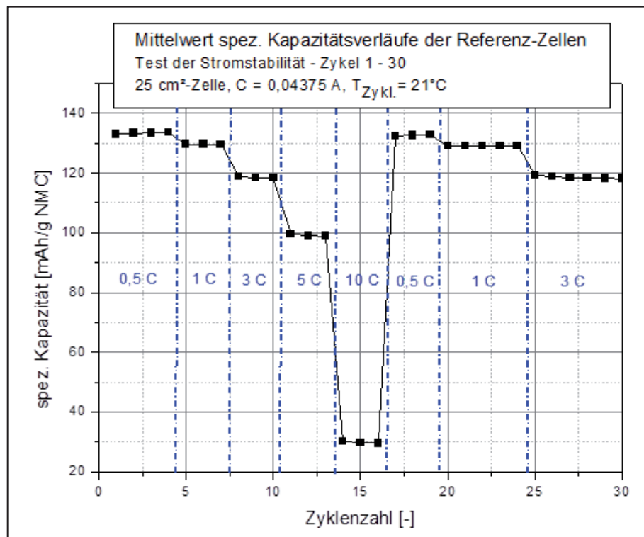
Abbildung C-7: Elektrochemischer Zyklentest einer Referenzzelle aus Neumaterialien – Charakterisierung der Stromstabilität bei variiert Laderate
