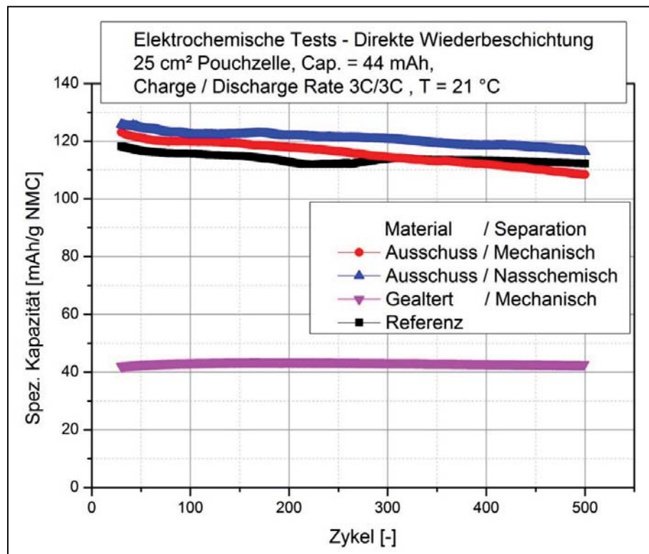
Abbildung C-8: Elektrochemische Kapazitätsverläufe von Referenz und zyklisierten Materialien
