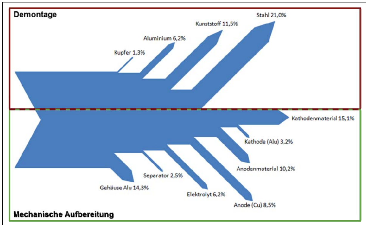
Abbildung G-3: Sankey-Diagramm zum Materialfluss in den Prozessen
