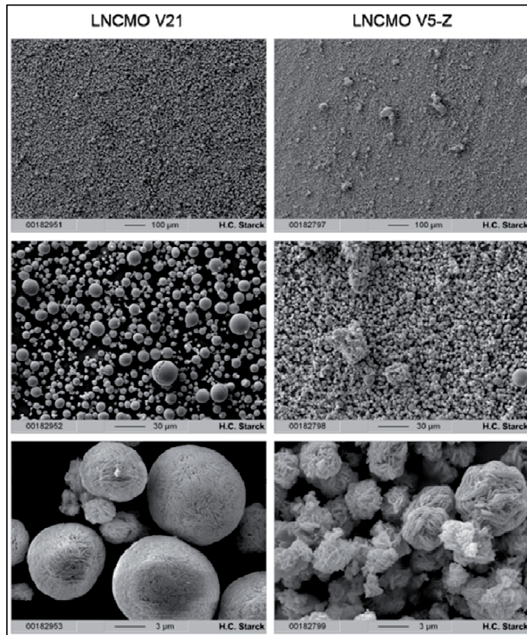
Abbildung C-2: REM-Aufnahmen der Precursor aus recycelten Lösungen bei 200-, 1.000- und 5.000-facher Vergrößerung
