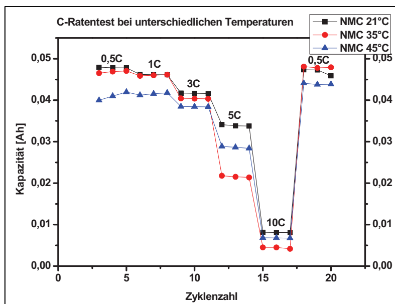
Abbildung D-12: C-Ratentest bei unterschiedlichen Temperaturen
