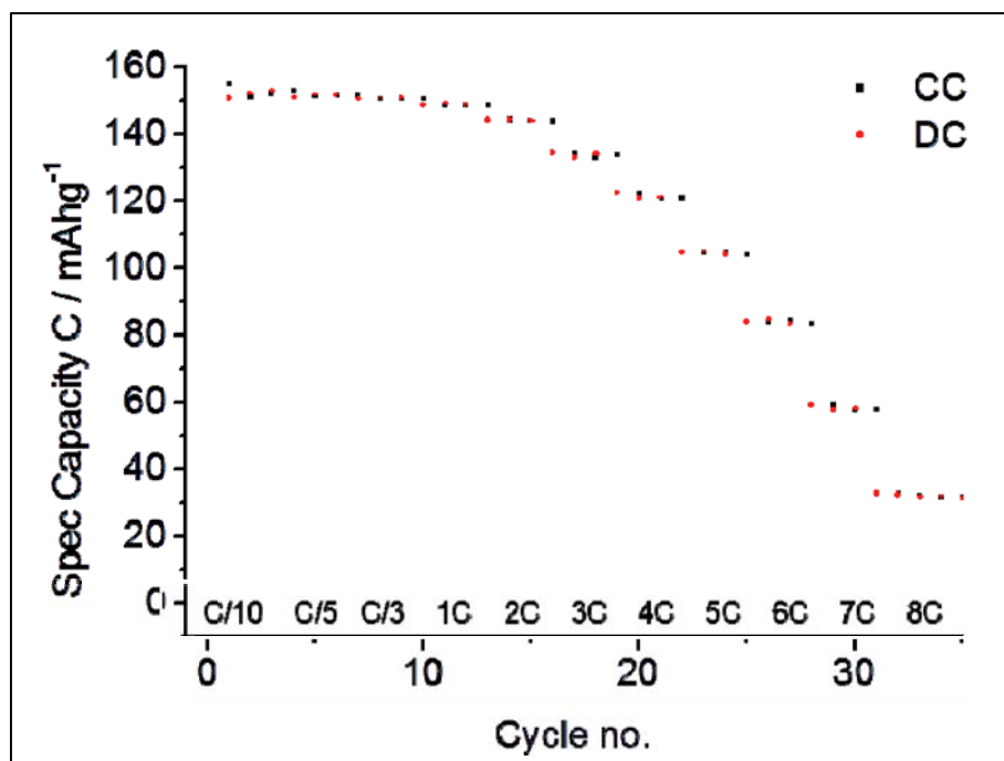
Abbildungung C-5: DC-Ratentest von LiBF 4 in EC/DMC
