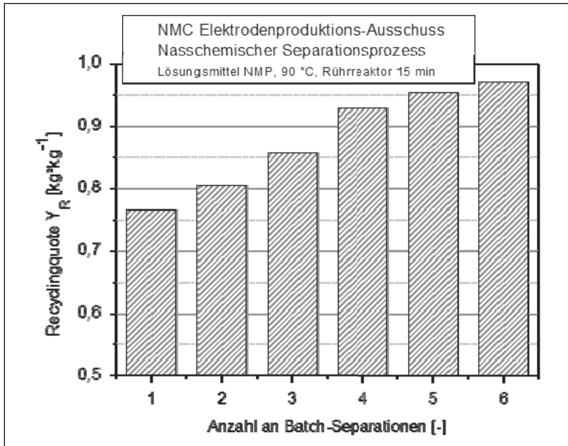
Abbildung B-25: Recyclingquote über Anzahl der Batch-Lösevorgänge
