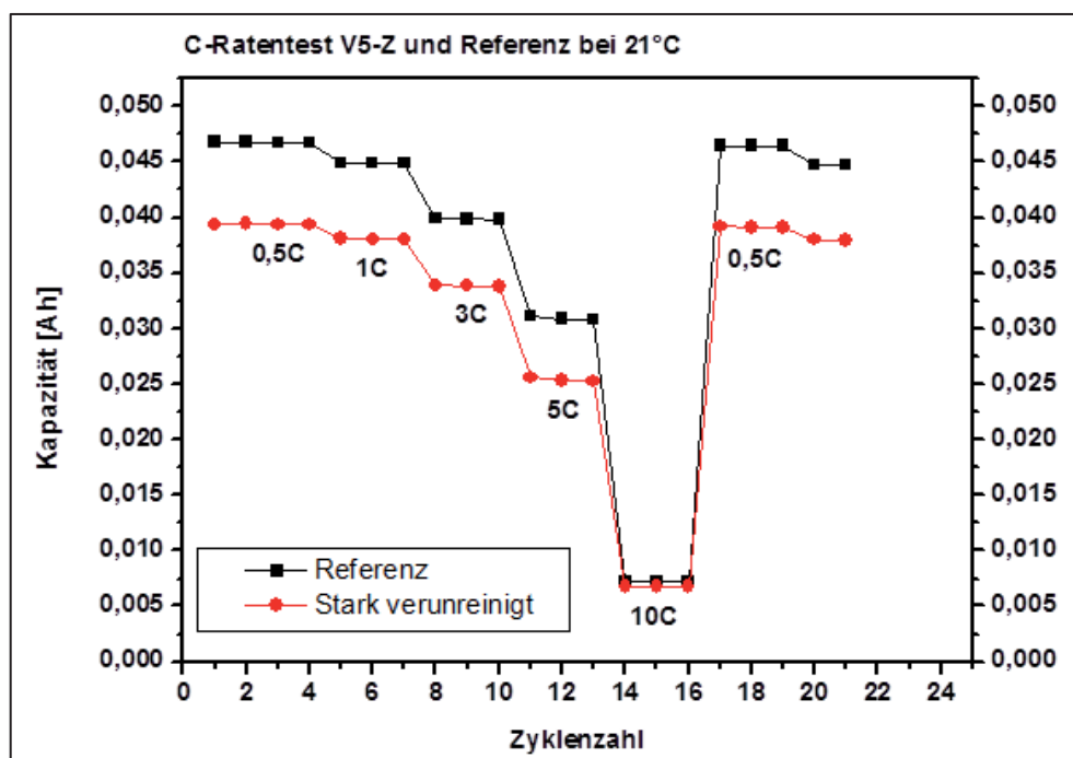
Abbildung C-19: C-Ratentest V5-Z und Referenz
