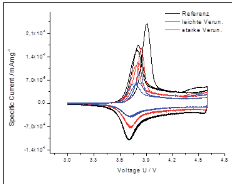
Abbildung C-17: CV Daten aller drei Materialien
