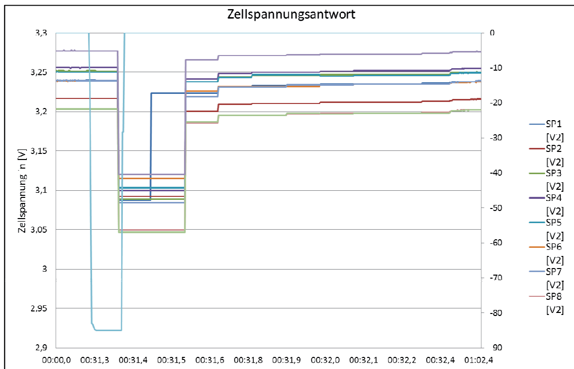
Abbildung D-8: Sprungantwort der Einzelzellspannungen
