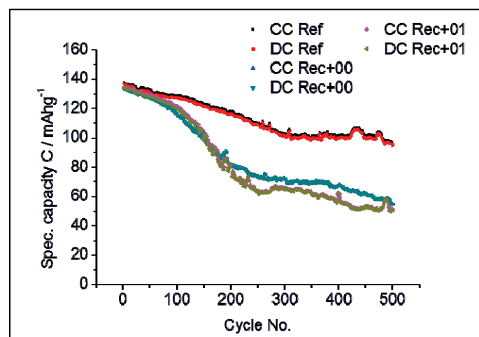
Abbildung D-2: Zyklisierungskurve von NMC bei 40°C
