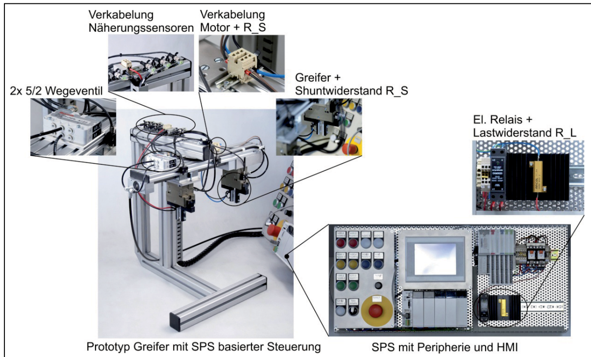
Abbildung B-14: Greifersystem mit einzelnen Subsystemen und Komponenten
