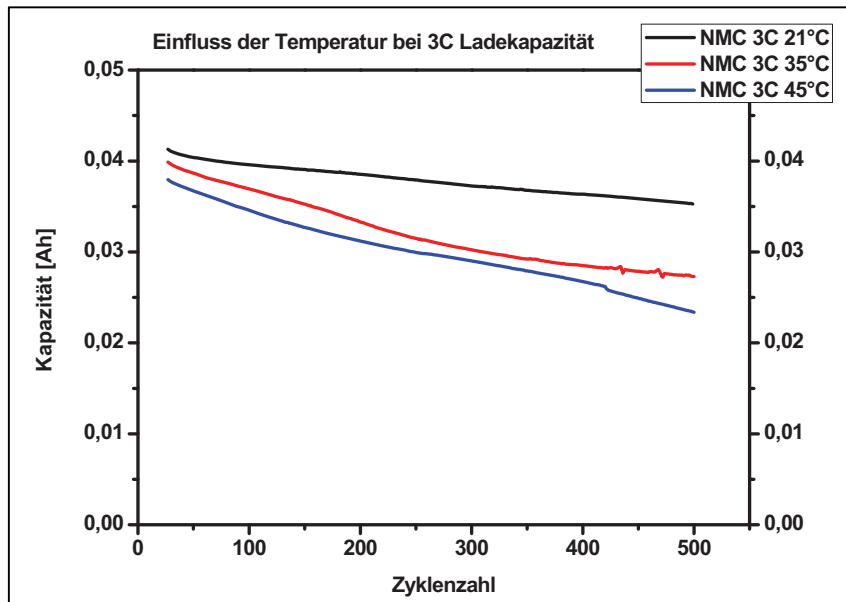
Abbildung D-11: Performance von Standard-Schichtoxid-Zellen bei 3C Laderate
