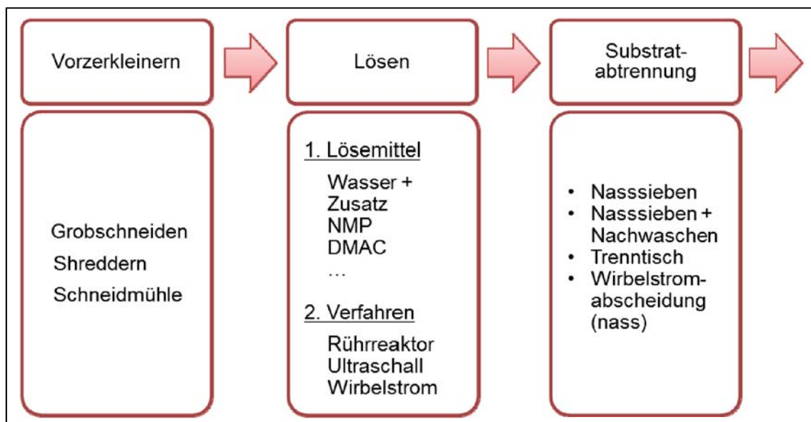
Abbildung B-27: Verfahrensfließbild zu Prozessalternativen der Nasschemischen Separation der Beschichtung von Batterie-Elektroden
