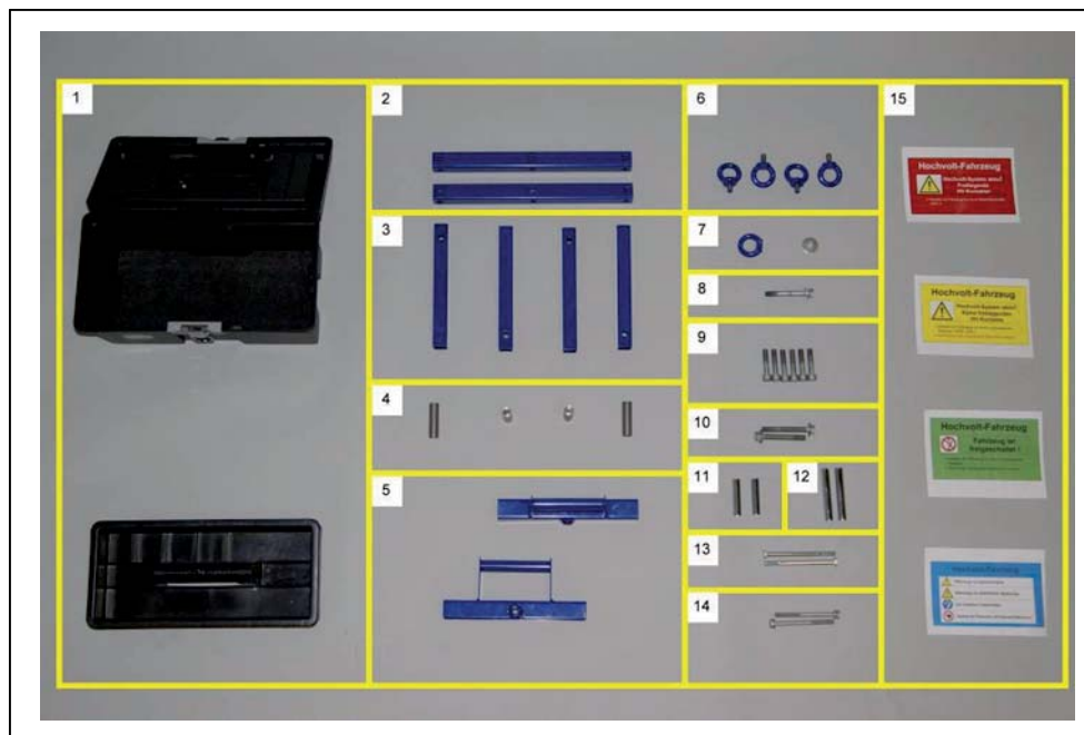
Abbildung A-10: HV - Batteriedemontage-KIT
