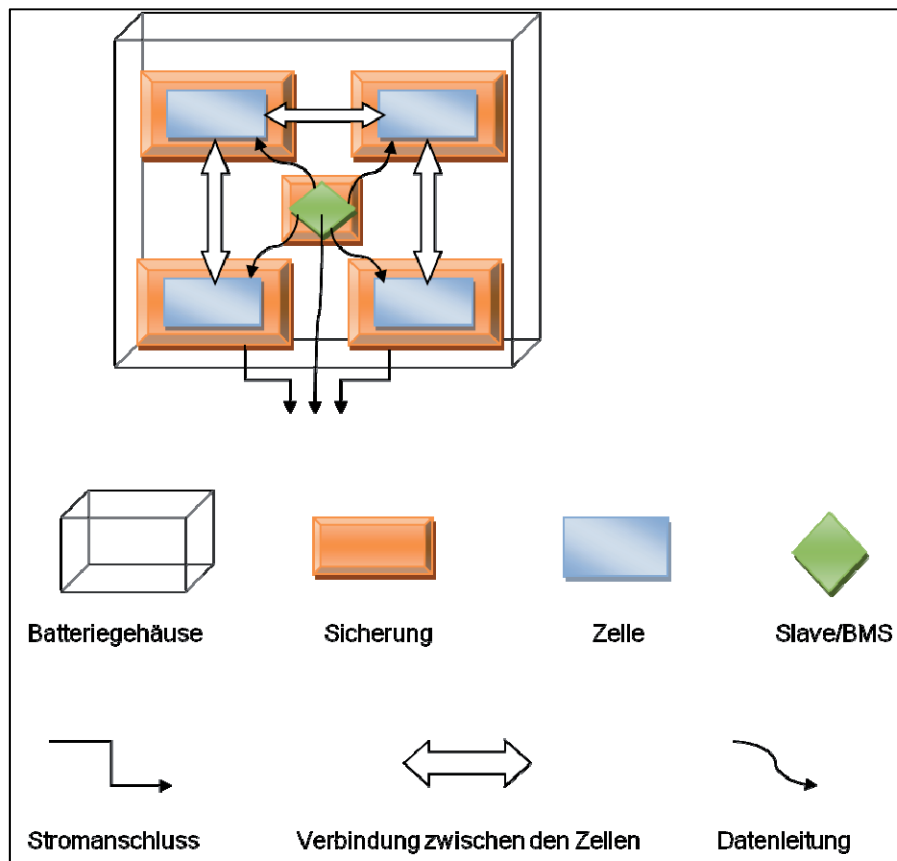
Abbildung F-4: Gesamtsystem Batterie mit allen notwendigen Komponenten
