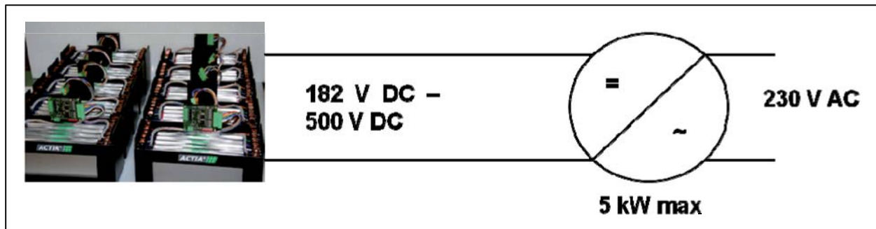
Abbildung A-23: Schematischer Aufbau des Entladeverfahrens von Batteriesystemen
