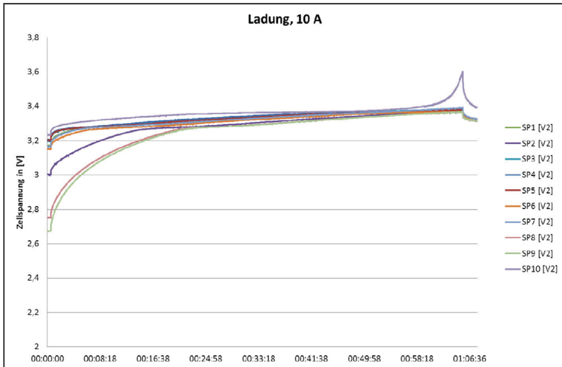
Abbildung D-6: Ladung der zu charakterisierenden Standardzellen
