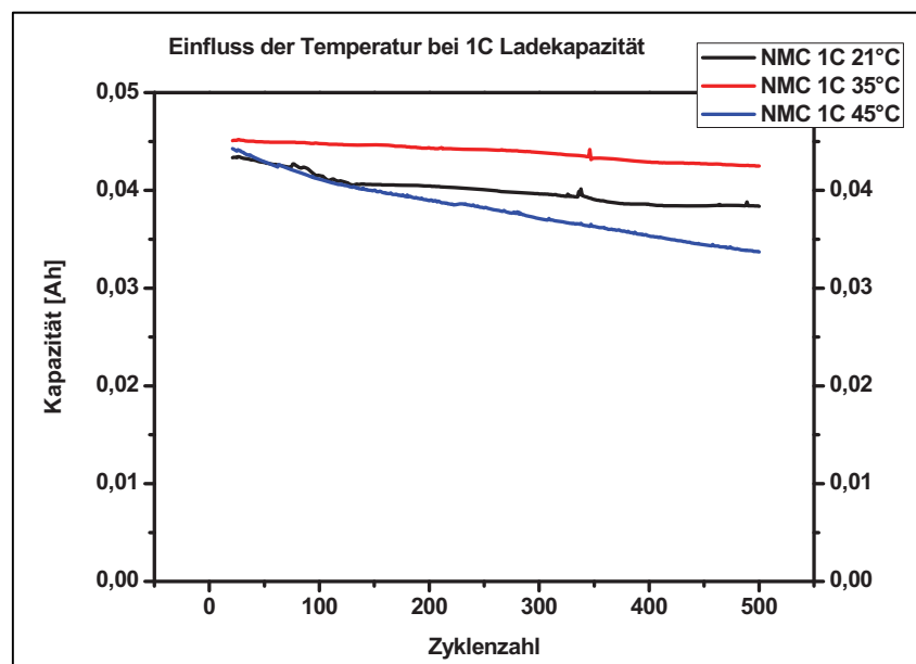
Abbildung D-10: Performance von Standard-Schichtoxid-Zellen bei 1C Laderate
