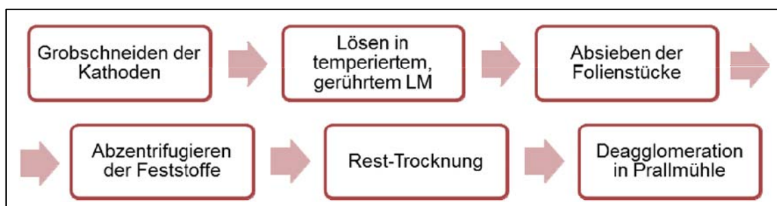
Abbildung B-24: Verfahrensfließbild Nasschemische Separation der Beschichtung von Batterie-Elektroden
