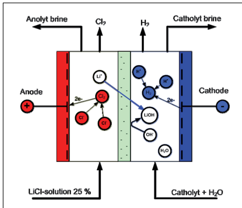
Abbildung B-33: Funktionsweise einer Elektrolyse mit monopolarer Membran
