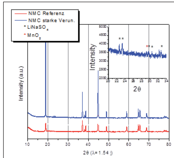
Abbildung C-15: XRD Messungen
