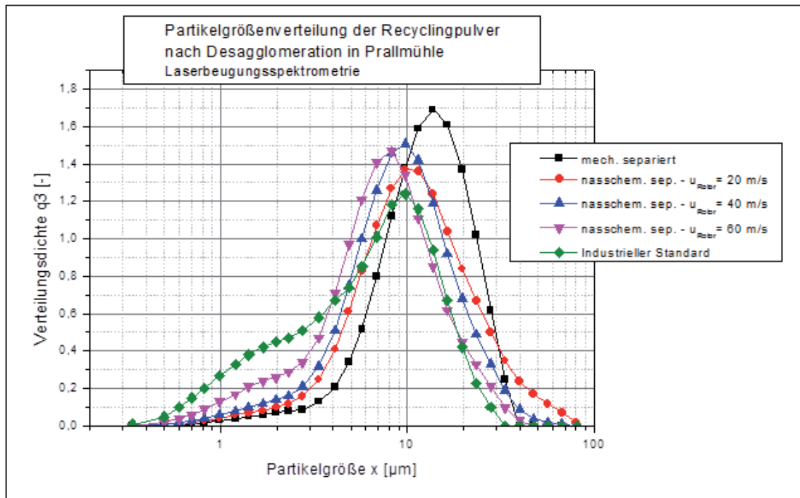
Abbildung B-28: Partikelgrößenverteilung der wiedergewonnenen Beschichtung nach Desagglomeration in Prallmühle
