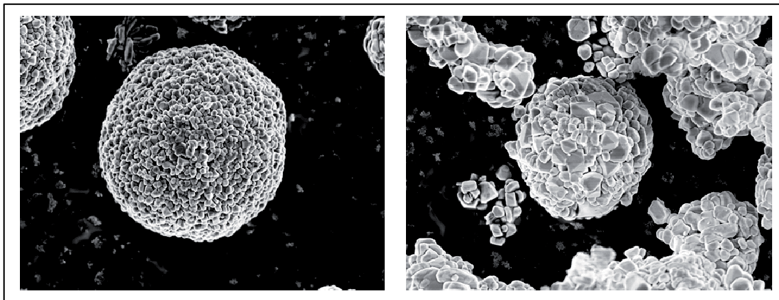
Abbildung C-16: Ansicht der Primärpartikel bei der Referenz (links) und starke Verunreinigung (rechts)
