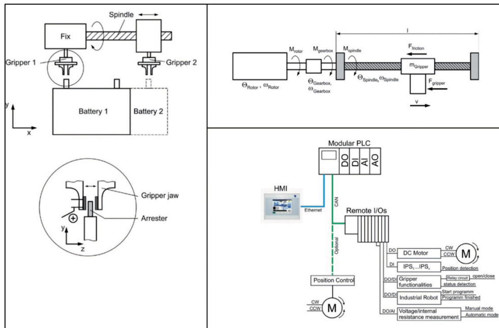
Abbildung B-9: Prinzip der Greifvorrichtung (links); Parameter zur Motorauslegung (oben rechts) und Steuerungsarchitektur (unten rechts)
