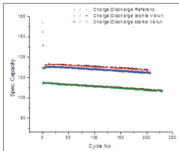
Abbildung C-18: Zyklenstabilität
