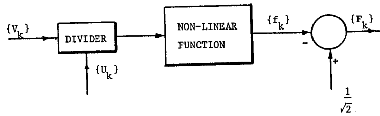
FIGURE 6.12 - The Non-Linear Element NEL.
