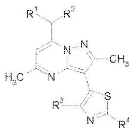
式 I
