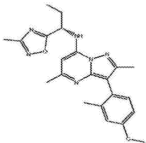
化合物 I
