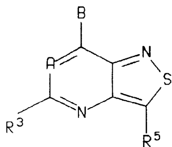
I - T
