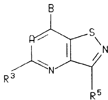
I - X
