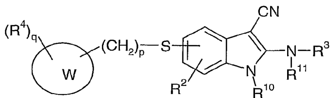
Formula (D)
