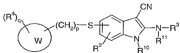
Formula (D)
