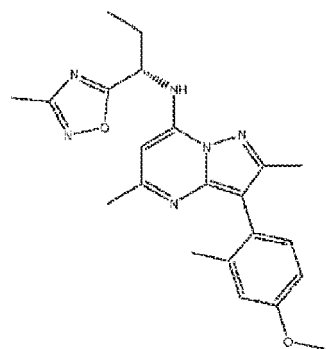
化合物I
