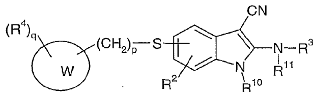
Formula (D)
