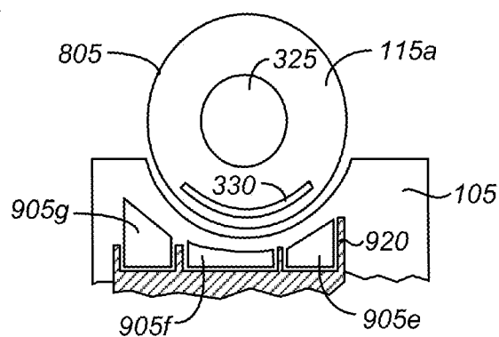
SECTION B-B FIG. 12
